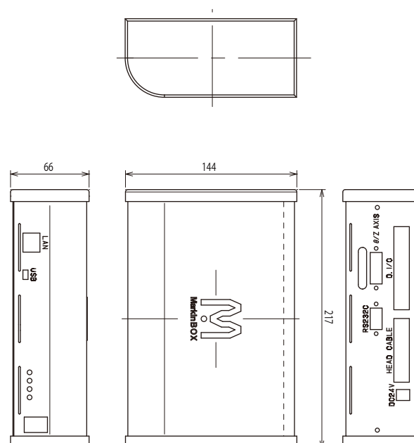
MB2Sコントローラ 外観図
