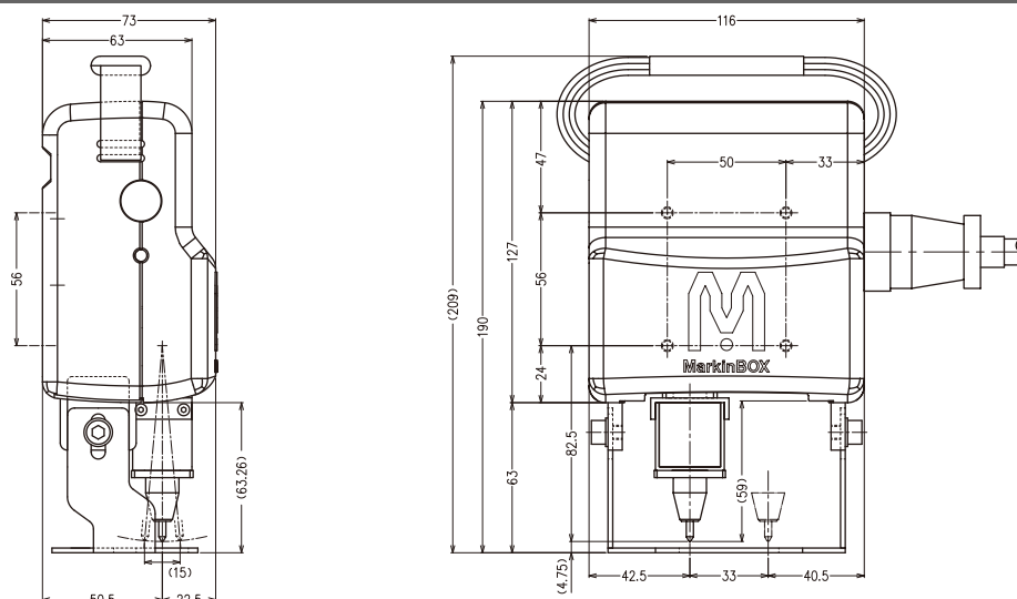
MB 3315S 外観図
