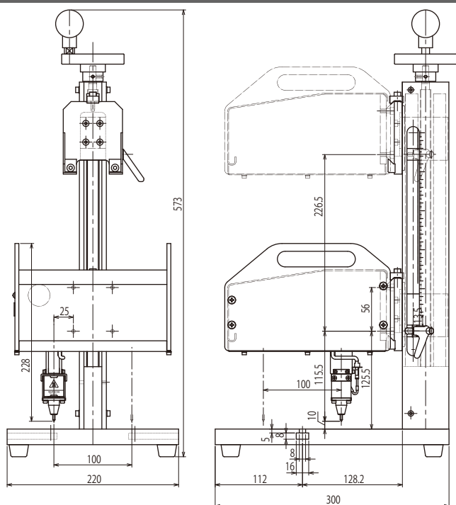
MB 1010 外観図
