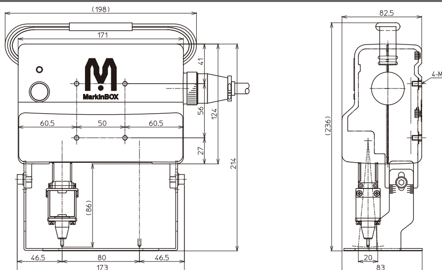
MB 8020S 外観図
